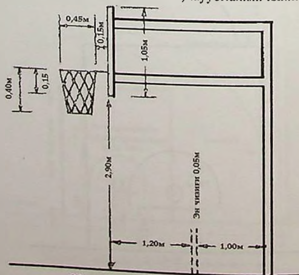
39-rasm. Halqa shit qurilmasi.
