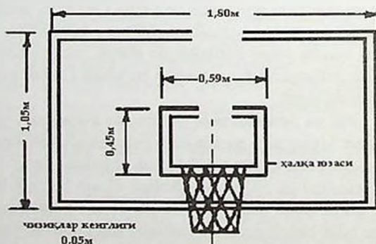
40-rasm. Shit. Uning o'lchovlari.
